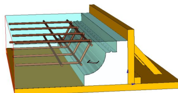
Coffrage sur plateau
